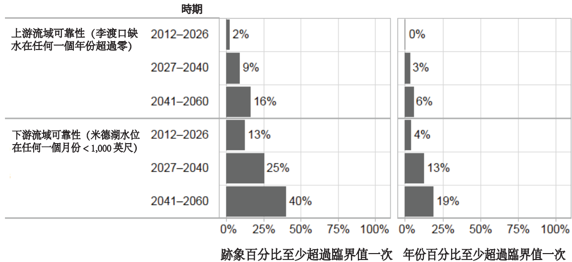
圖 S. 1 未達目標的長期供水結果摘要
