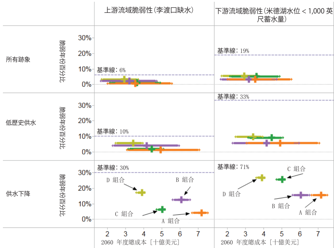
圖 S. 2 上游和下游流域的各種組合間的組合成本與脆弱性 (2041 - 2060) 的對比取捨
